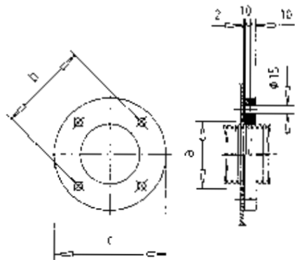
Schienen / Barres / Busbars – Ø 55 / 67 / 80 / 106
