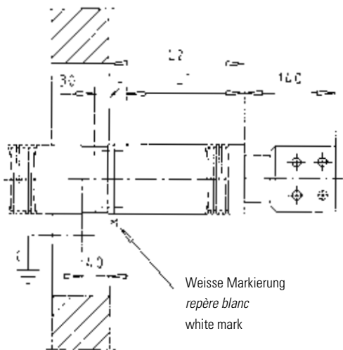
Schienen / Barres / Busbars – Ø 55 / 67 / 80 / 106
