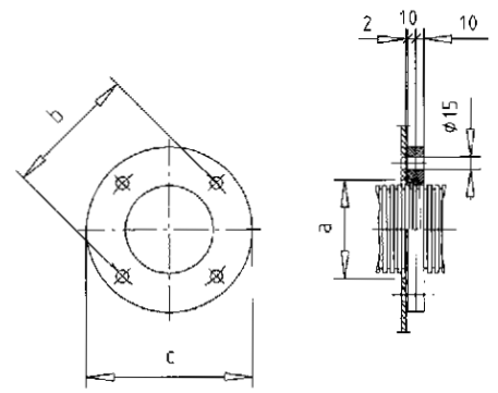
Schienen / Busbars – \phi 55 / 67 / 80 / 106
