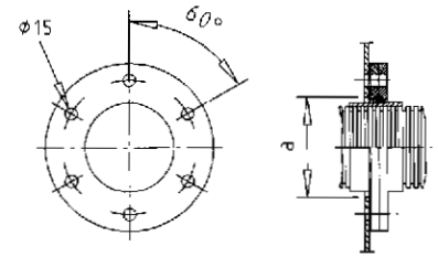
Schienen / Busbars – \phi 146
